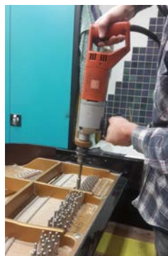
Abbildung 7: Ausdrehen der alten Wirbel (Stimmnägeln) an einem Klavier © Striegel
